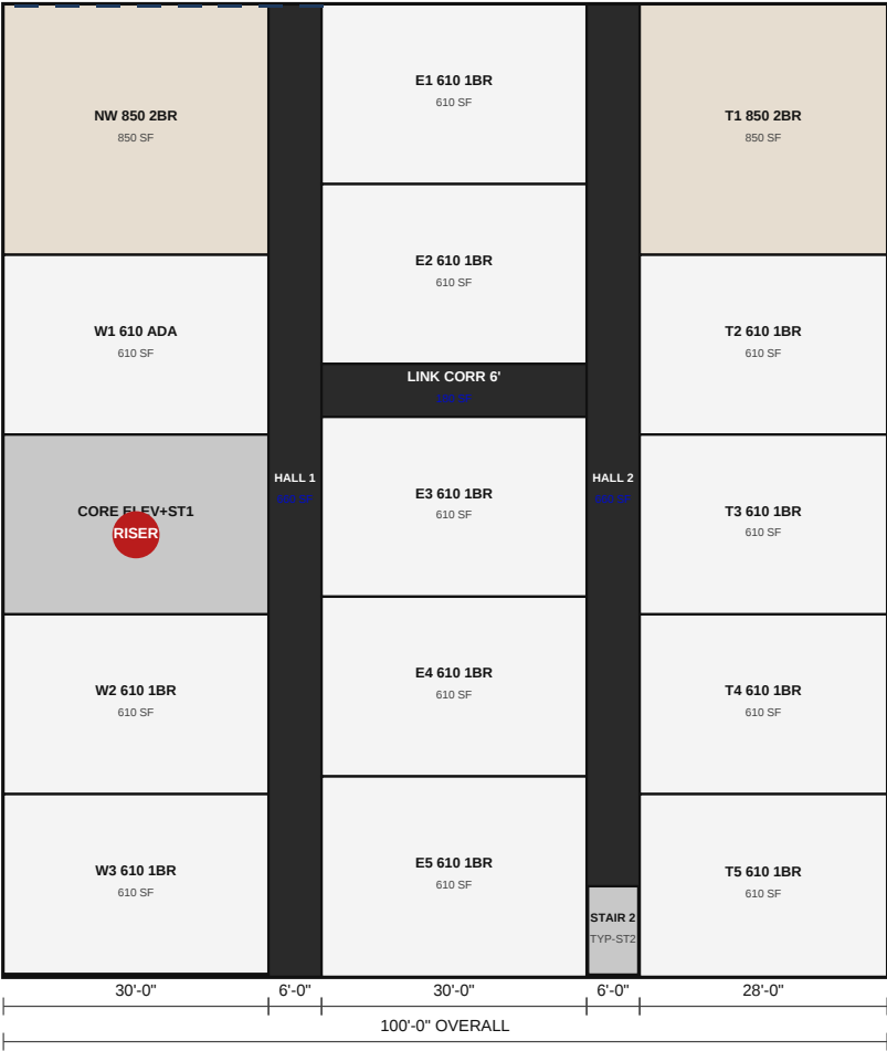
TYP FLOOR PLAN · 14 KEYS · FF 12'-0" 12×610 + 2×850 · HALLS & LINK 6'-0" · PACK 30+6+30+6+28 · LAYOUT LOCK Jul 12
